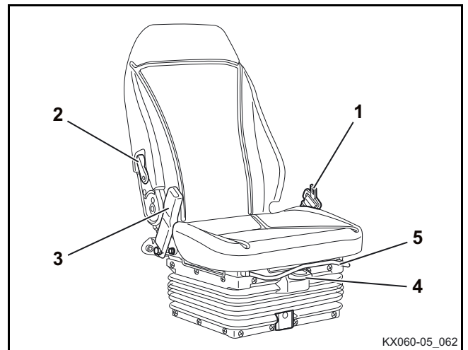
Luftgefederter Sitz (optional)
