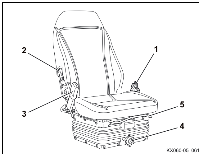
Mechanisch gefederter Sitz
